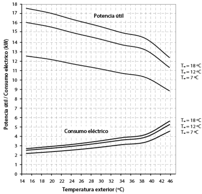
Curvas de prestaciones en enfriamiento Dual Clima 16HT/16HTT
