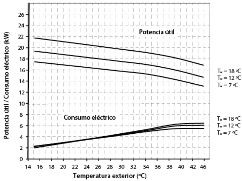
Curvas de prestaciones en enfriamiento Dual Clima 19HT/19HTT
