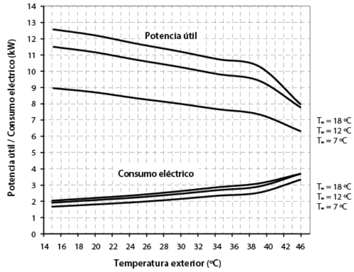
Curvas de prestaciones en enfriamiento Dual Clima 12HT/12HTT
