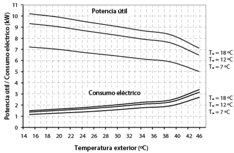
Curvas de eficiencia en enfriamiento Dual Clima 9HT (EER)
