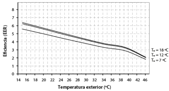
Curvas de eficiencia en enfriamiento Dual Clima 16HT/16HTT (EER)
