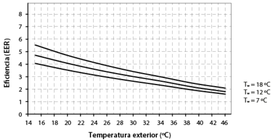
Curvas de eficiencia en enfriamiento Dual Clima 22HTT (EER)
