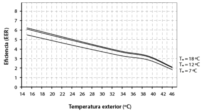
Curvas de eficiencia en enfriamiento Dual Clima 12HT/12HTT (EER)
