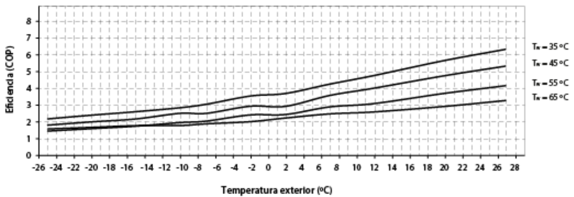
Curvas de eficiencia en calentamiento Dual Clima 16HT/16HTT (COP)
