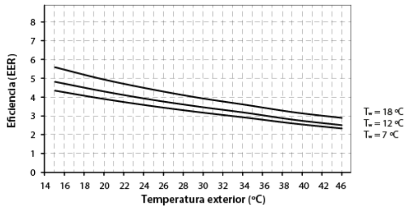
Curvas de eficiencia en enfriamiento Dual Clima 19HT/19HTT (EER)
