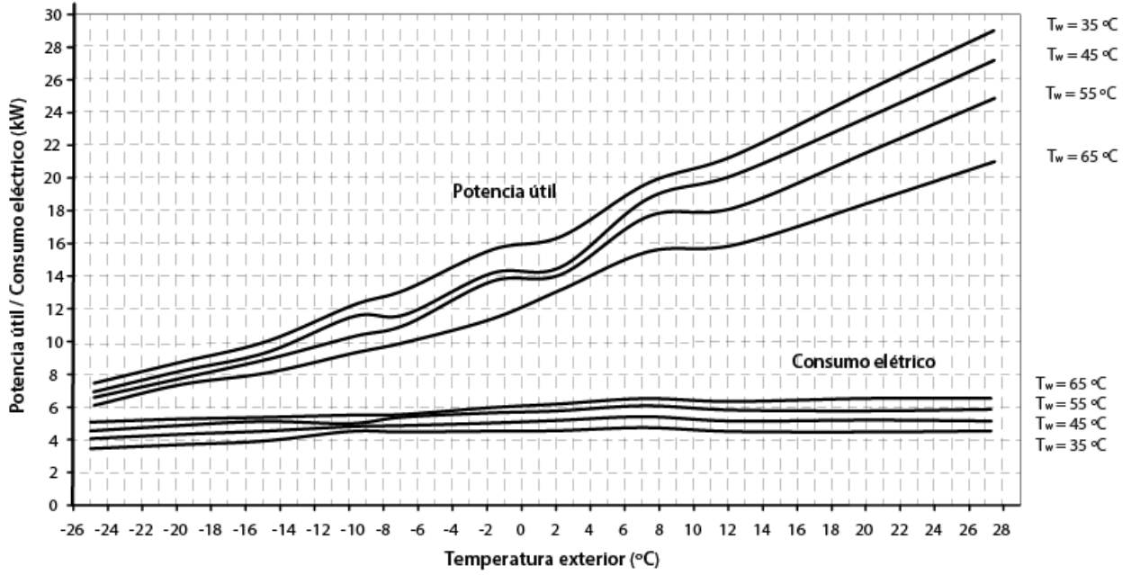
Curvas de prestaciones en calentamiento Dual Clima 19HT/19HTT
