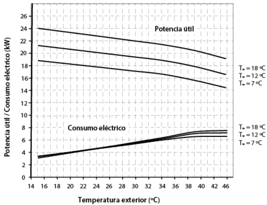
Curvas de prestaciones en enfriamiento Dual Clima 22HTT
