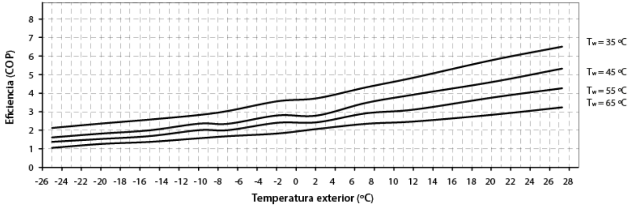
Curvas de eficiencia en calentamiento Dual Clima 19HT/19HTT (COP)
