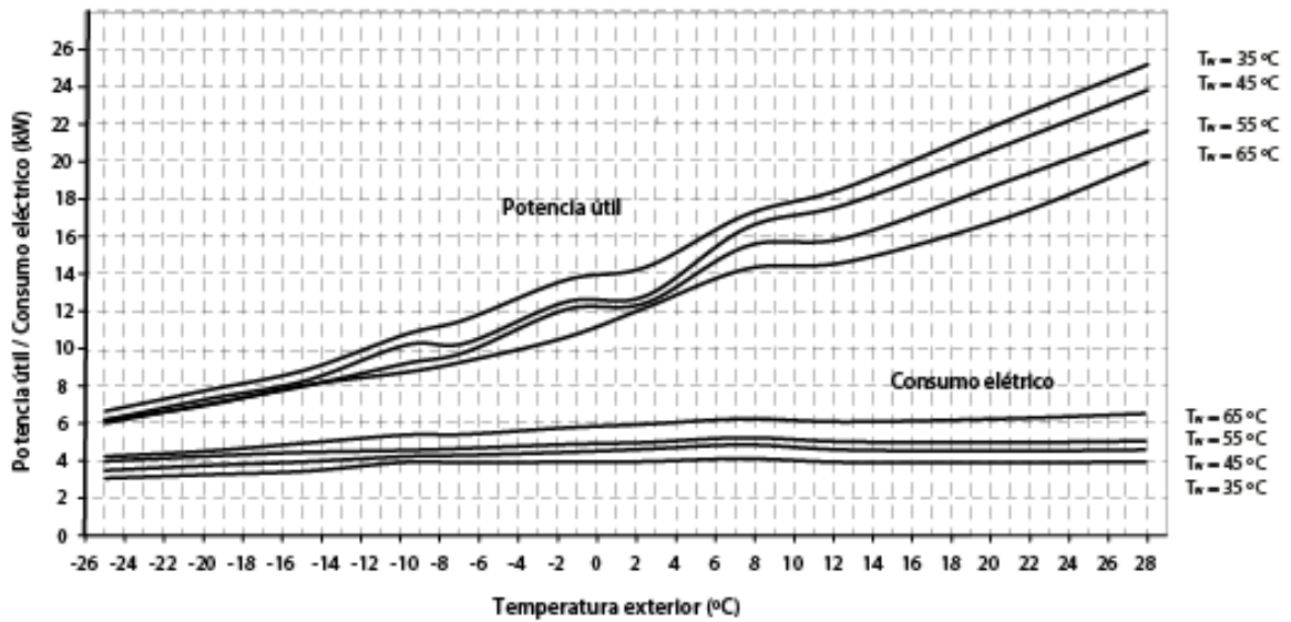
Curvas de prestaciones en calentamiento Dual Clima 16HT/16HTT
