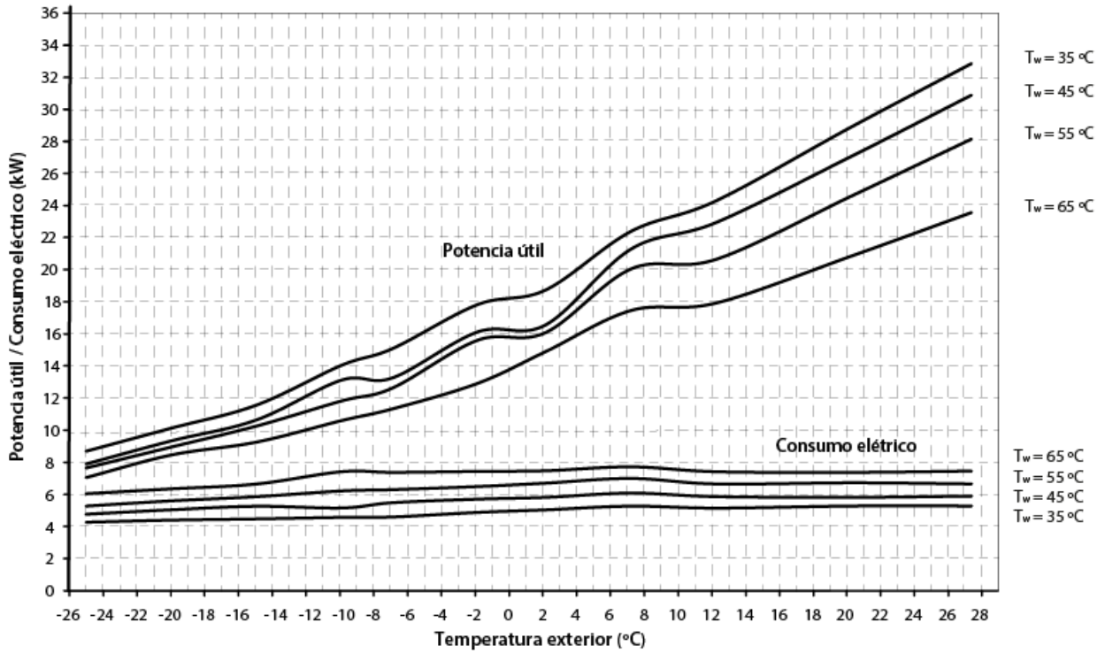
Curvas de prestaciones en calentamiento Dual Clima 22HTT
