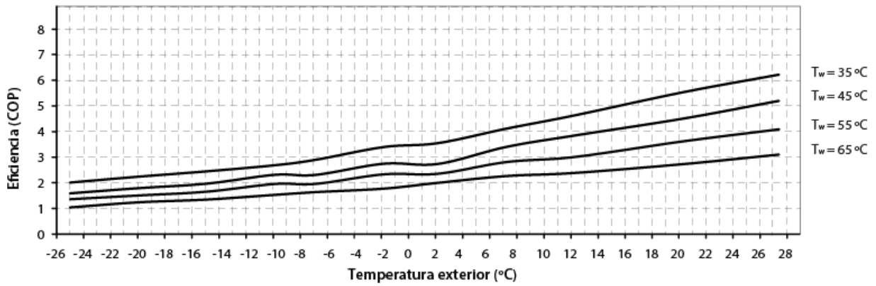
Curvas de eficiencia en calentamiento Dual Clima 22HTT (COP)
